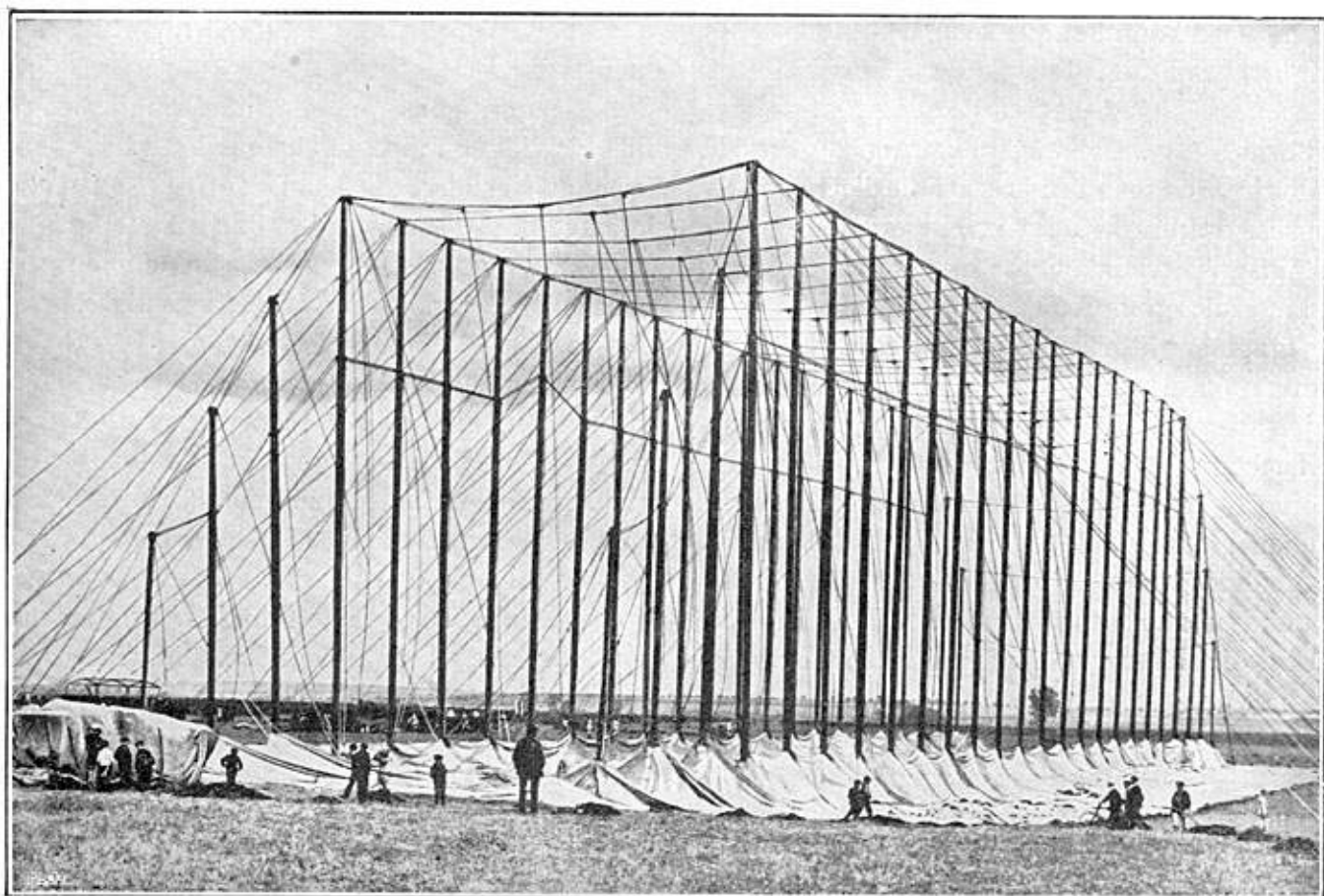
LE MONTAGE D'UN HANGAR DE ZEPPELIN
