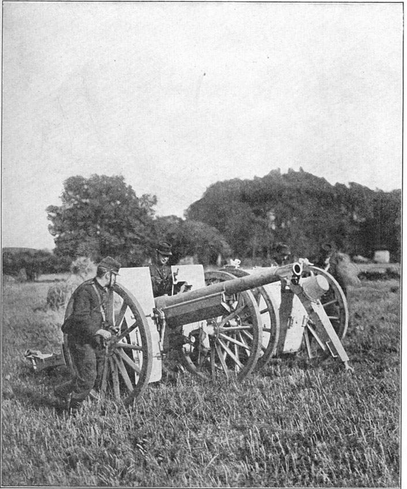
LE CANON FRANÇAIS DE 75
